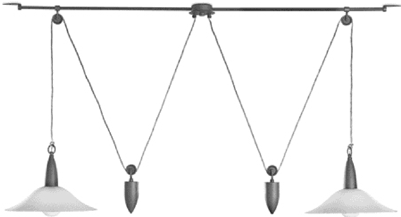
2322.02P 2 luci - Piombo Ø 35 L. max 170 L. min 85 cm. E27#2x60W
